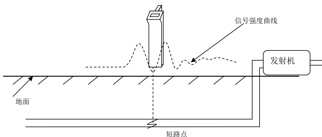
线间短路测试示意图
