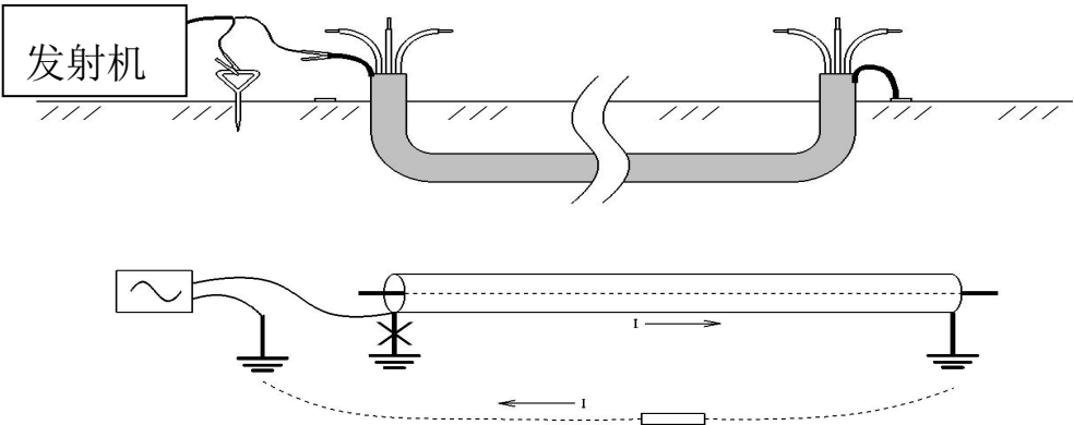
图 4. 2 护层—大地接线法
