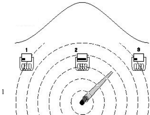
波峰法原理
