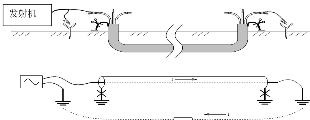
图 4.1 芯线-大地接线法
