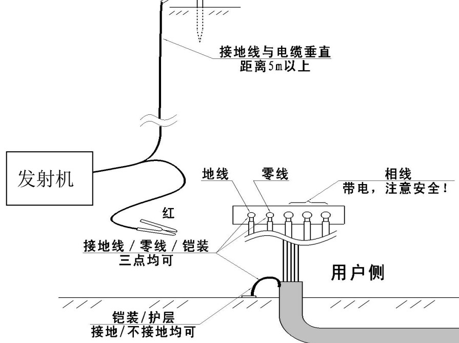
图 4.6 零线 / 地线 / 护层注入法
