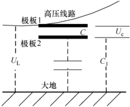
图 3-1 电场空间取电原理图
