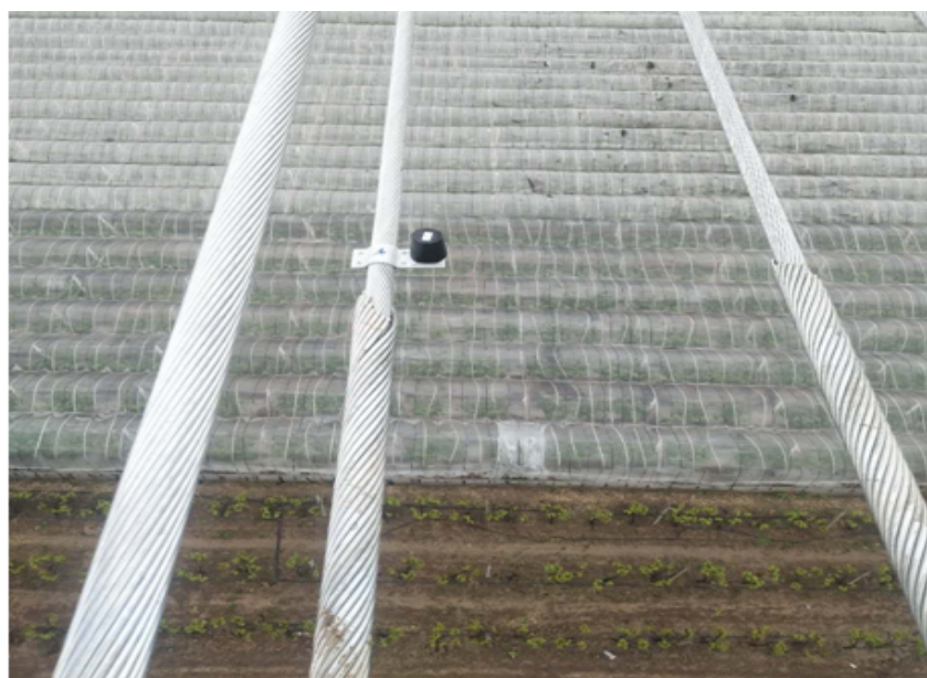
安装在 500kV 输电线路
