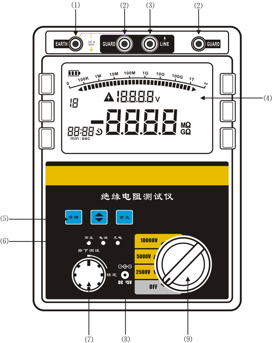
图 1：YTC2303 面板结构说明
