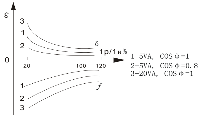
电流互感器的负荷特性曲线
