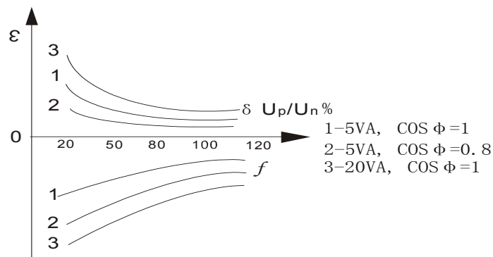
电压互感器电压与负荷特性
