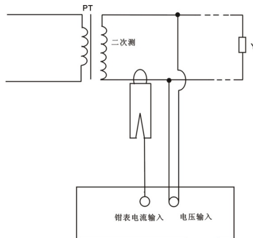
单相 PT 负荷测试接线图
